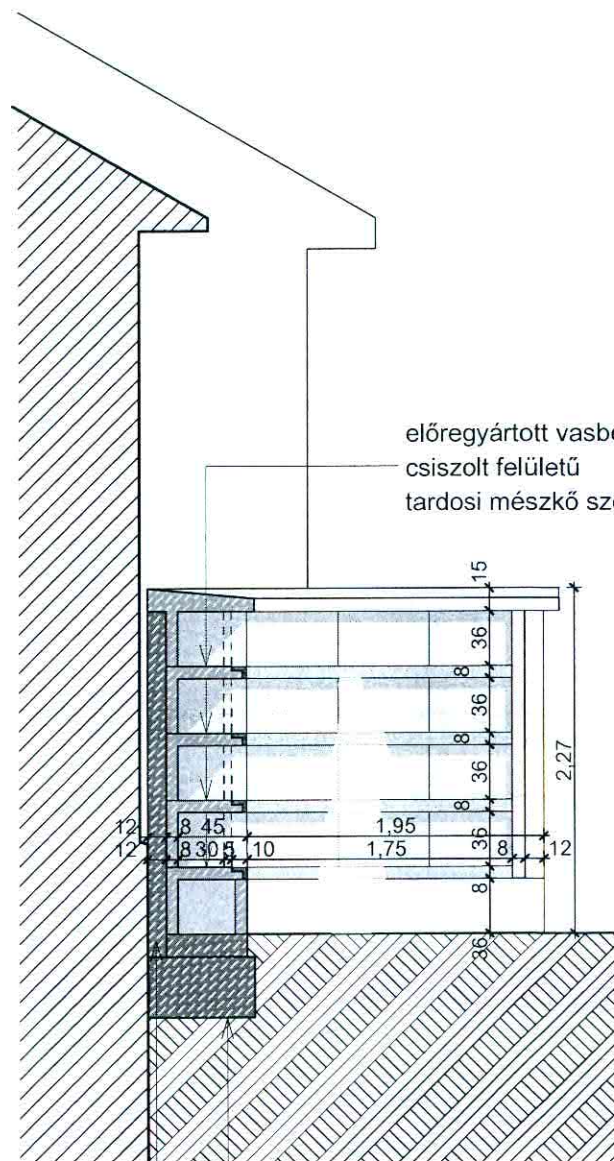
A-A metszet
