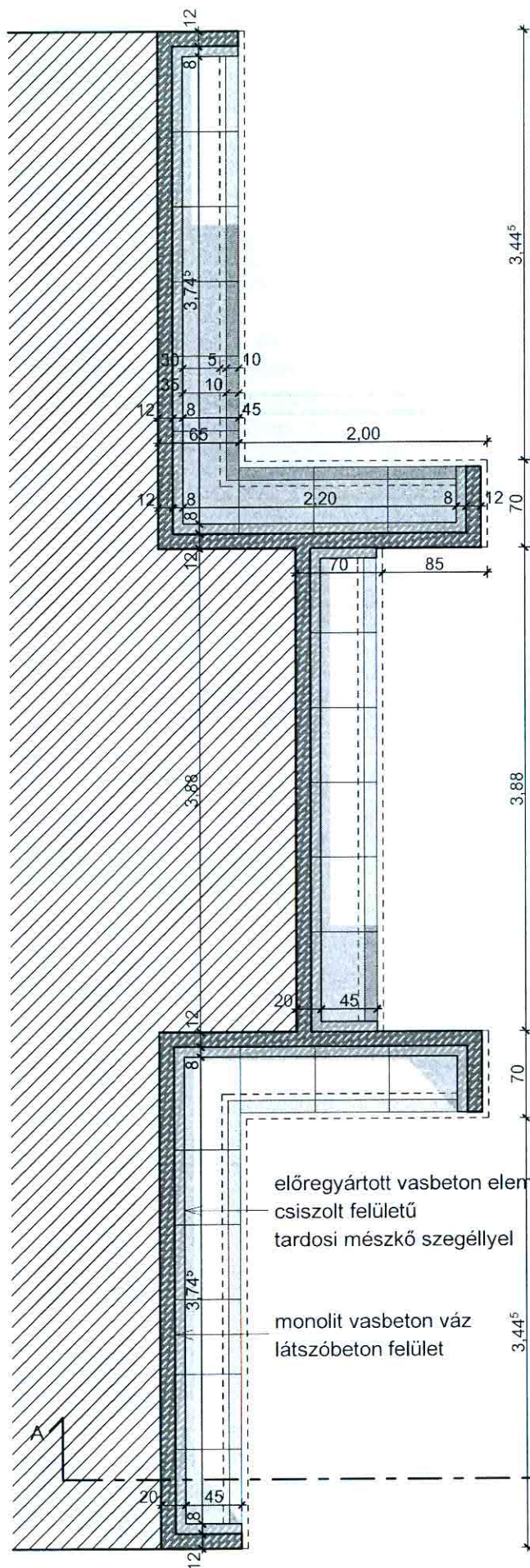
A-A metszet
